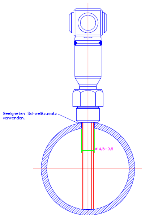
DF12 mit Schneidringstutzen
