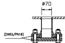
Gegenlager DF50 Seite 6 / Kapitel 6 Opposite support DF50 Page 6 / Chapter 6
