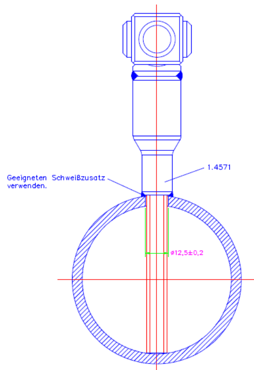
DF12 Einschweißversion
